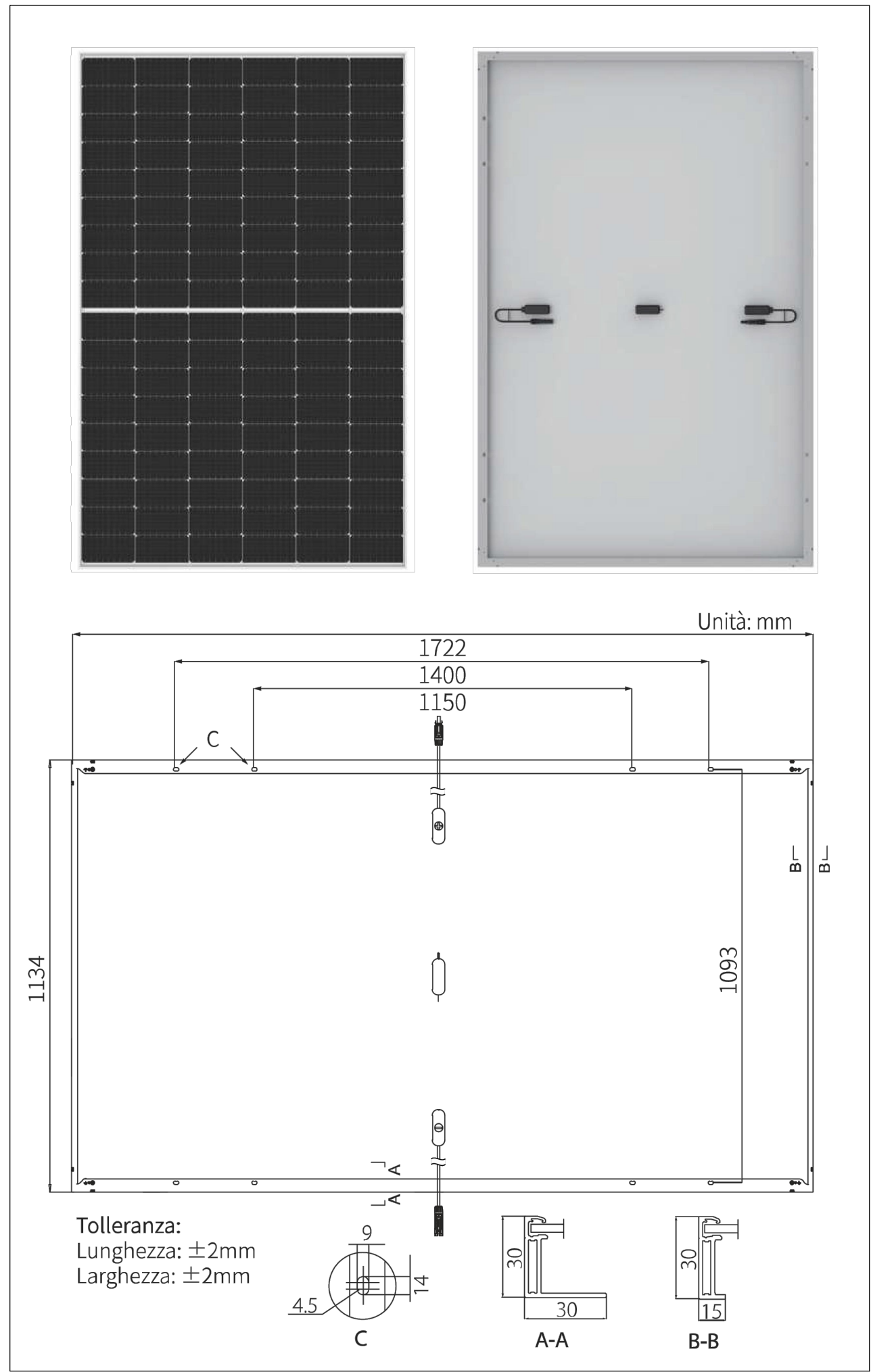
PARTICOLARE PANNELLO FOTOVOLTAICO
